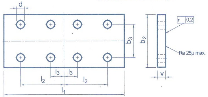
标准连接板 Standard fishplate.
